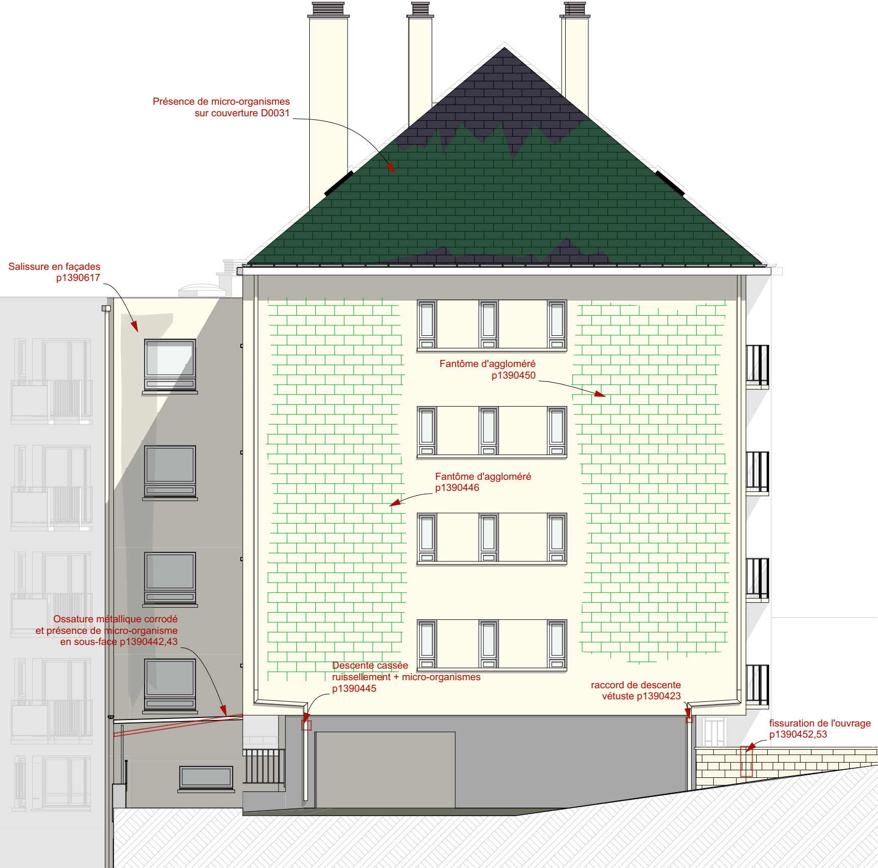
Nord/Ouest Façade N/O (1) 1:100
