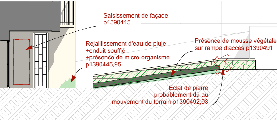
Descente Nord/Ouest Descente N/O 1:100
